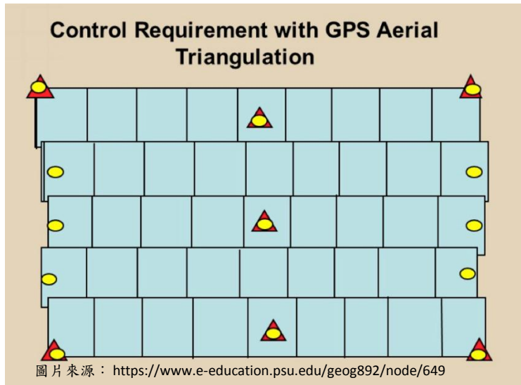
地面控制點規劃佈設方式
